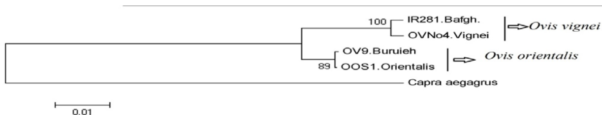
شکل ۵- درخت فیلوژنتیک قوچ بر اساس توالی‌های سیتوکروم b
