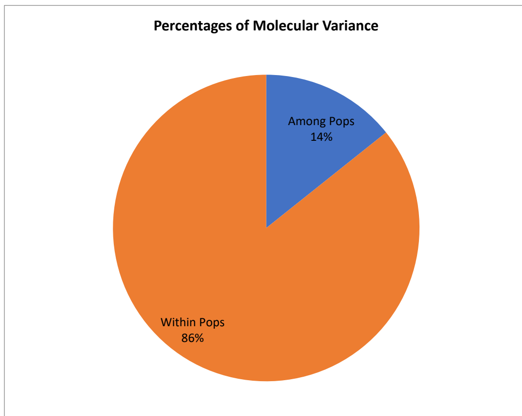
شکل ۳. تجزیه واریانس مولکولی در جمعیت‌های هندوانه مورد مطالعه
