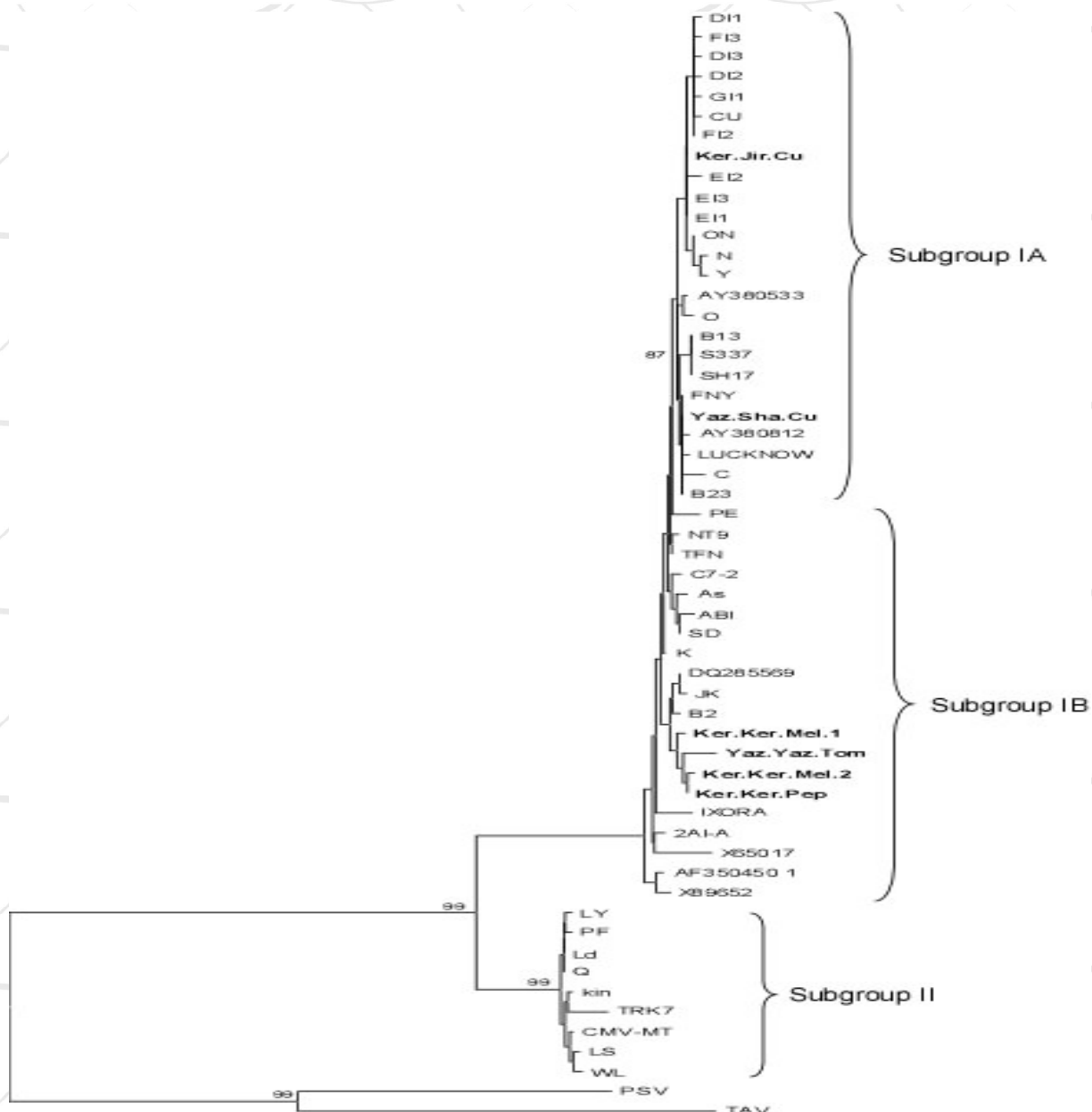
شکل 4- درخت فیلوژنتیکی رسم شده بر اساس روش neighbor-joining با استفاده از نرم افزار MEGA 4 بر پایه ترادف اسیدهای آمینه پروتئین پوششی جدایه های ایرانی ویروس CMV و سایر جدایه های موجود در بانک ژن. جدایه های ایرانی مورد بررسی در این تحقیق به صورت Bold نشان داده شده اند. جدا یه ای از TAV به نام AJ237849.2 و جدایه ای از PSV به نام NC_002040 به عنوان Outgroup انتخاب گردیده اند.
