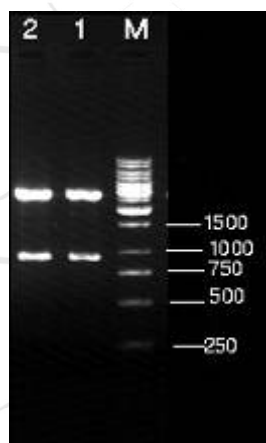
شکل 2 - الکتروفورز پلاسمید نو ترکیب حاوی قطعه ژن پروتئین پوششی جدایه های ایرانی TAV هضم شده با آنزیم های EcoR1 و Pst1 درون ژل آگاروز 1% (M نشانگر اندازه 1Kb DNA (Gen Ruler™ DNA Ladder, Fermentase). (1) جدایه Ker.Jir.Cu. متعلق به زیر گروه IA. (2) جدایه Yaz.Yaz.Tom متعلق به زیر گروه IB.
