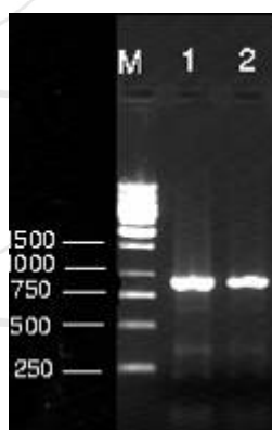
شکل 1- الکتروفورز محصول PCR تکثیر شده با استفاده از آغازگرهای اختصاصی R-DAG/F-DAG و تشکیل باند 946 جفت بازی مربوط به ژن پروتئین پوششی جدایه‌های ایرانی CMV درون ژل آگاروز 1%. (M نشانگر اندازه DNA (Gene Ruler™1Kb DNA Ladder، DNA اندازه Fermentase). جدایه Ker.Jir.Cu. متعلق به زیر گروه IA. 2) جدایه Yaz.Yaz.Tom متعلق به زیر گروه IB.
