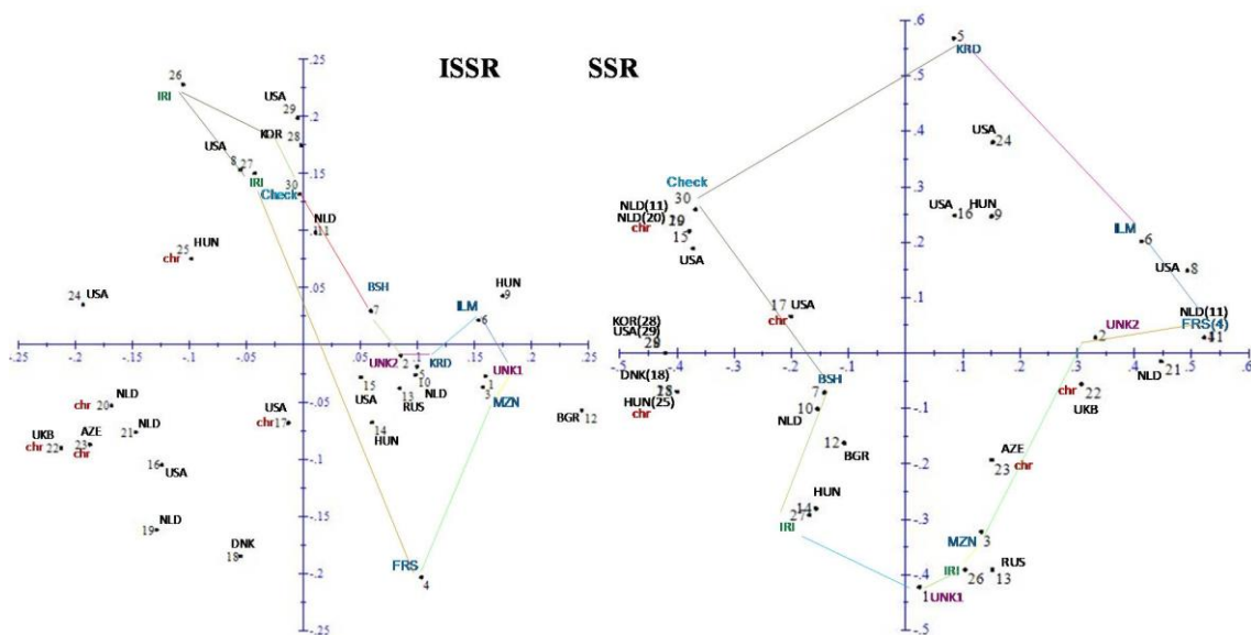
شکل ۵. توزیع توده‌های گوجه فرنگی ایرانی مورد بررسی بر اساس نمودار بای پلات حاصل از تجزیه به مختصات اصلی با استفاده از نشانگرهای ISSR (سمت چپ) و SSR (سمت راست)
