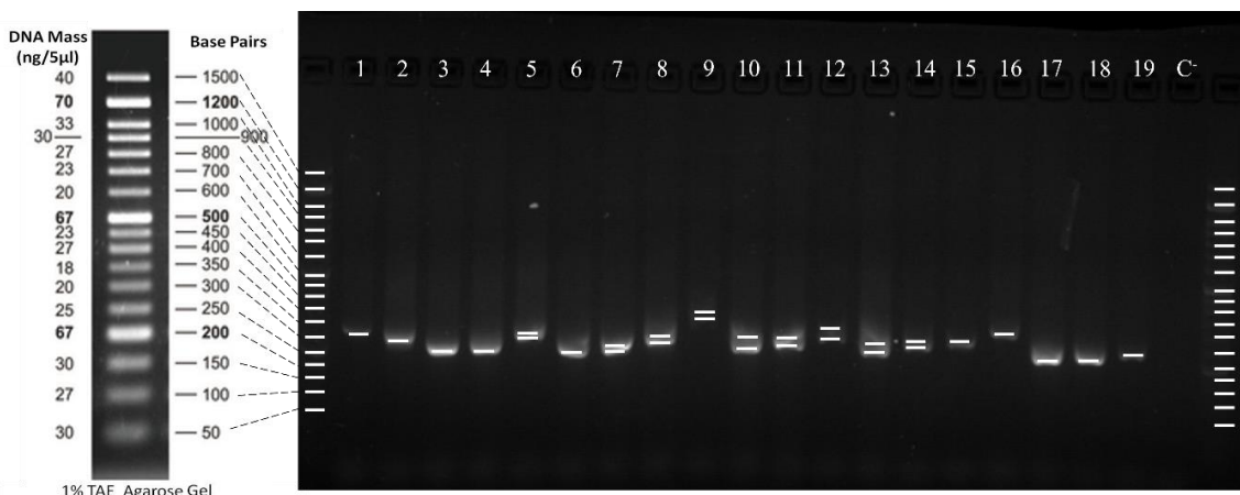
شکل ۱. الگوی بانندی توده های گوجه فرنگی مورد مطالعه بر اساس آغازگر (A) ISSR-3 و آغازگر (B) SSR-63F.
