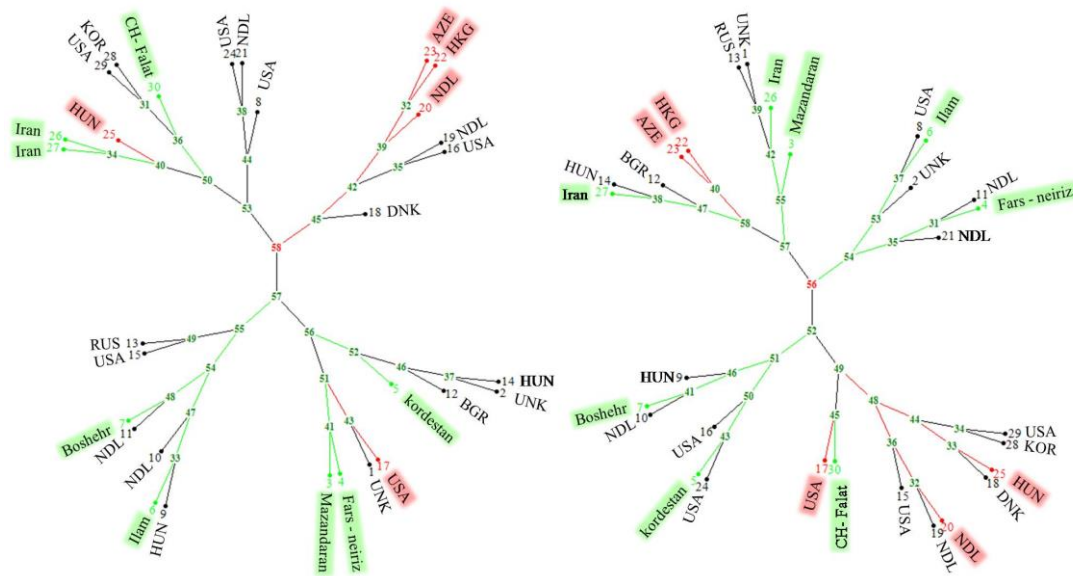
شکل ۳. تجزیه خوشه‌ای توده‌های گوجه فرنگی با استفاده از آغازگرهای ISSR (سمت چپ) و SSR (سمت راست) بر اساس ضرایب جاکارد و روش Neighbor-joining. توده‌های جمع‌آوری شده از مناطق مختلف ایران به رنگ سبز، توده‌های S. lycopersicum cherry با رنگ قرمز و توده‌های متعلق به S. lycopersicum esculentum با رنگ سیاه نشان داده شده است
