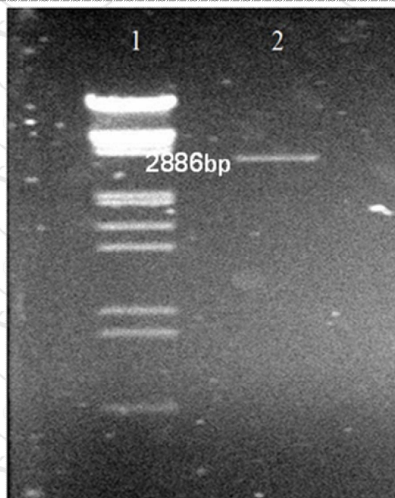
شکل 3- الکتروفورز پلاسمید pTZ57R برش یافته با آنزیم EcoRV پس از خالص سازی، در آگارز 1/2% (ستون 2) در کنار مارکر ژنوم لامبدا برش یافته با EcoRI و HindIII (ستون 1).
