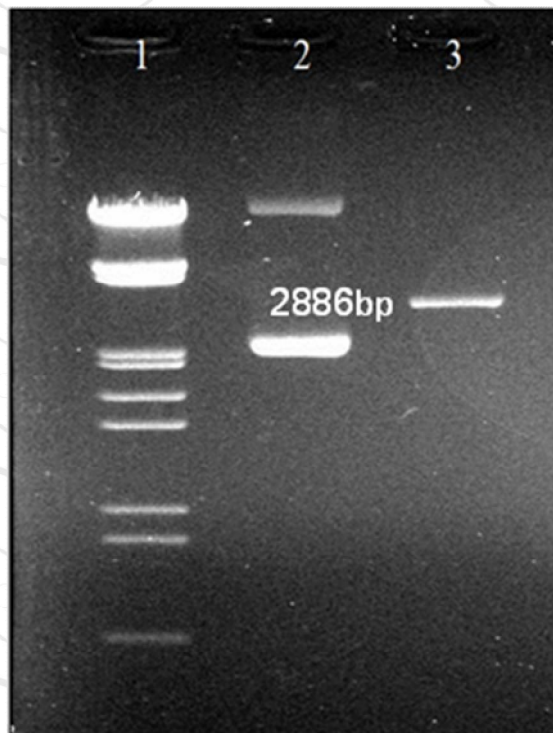
شکل 2- پلاسمیدهای استخراج شده از سلول‌های E. coli ترانسفورم شده با pTZ57R و الکتروفورز قطعه حاصل از برش آن با HindIII در آگارز 1/2%. ستون 1: ژنوم لامبدا برش یافته با EcoRI و HindIII . ستون 2: پلاسمید pTZ57R استخراج شده. ستون 3: پلاسمید pTZ57R استخراج شده بعد از برش با آنزیم HindIII
