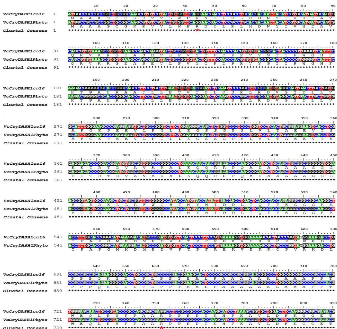
شکل ۴. بررسی شباهت توالی کدکننده ژن کریپتوکروم DASH1 ولوکس، حاصل از تعیین ترادف ( VcCryDASH1co16 ) و بازیابی شده از پایگاه داده‌های فیتوزوم ( VcCryDASH1Phyto )، با استفاده از همدریف‌سازی. در پایین هر توالی، اسیدهای آمینه‌ی به‌رمز در آمده، نشان داده شده است. همچنین شباهت نوکلوتیدی در ردیف "Clustal Consens" توسط علامت "*" تعیین شده است. علامت "*" قرمز رنگ، محل کدون نادر AGG را در توالی ژن VcCryDASH1 نشان می‌دهند.
