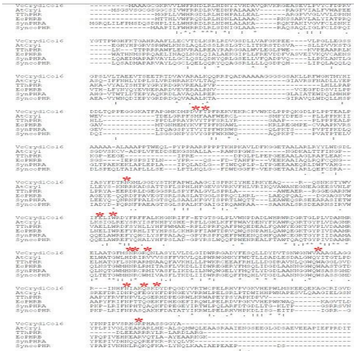
شکل ۹. هم‌ردیف‌سازی پروتئین‌های شاخص درون خانواده پروتئینی کریپتوکروم/فتولیزاز که قابلیت اتصال به DNA را دارند (پروتئین های TThPHR, EcPHRB, SynPHRA و SyncoPHR) و پروتئین شاخص درون این خانواده که قابلیت اتصال به DNA را ندارد (AtCry1)، با VcCryDASH1co16 به کمک الگوریتم Clustal omega. پروتئین‌های استفاده شده و ارگانیزم حاوی پروتئین در ادامه آورده شده است: TThPHR (Thermus thermophilus Deoxyribodipyrimidine photo-lyase)؛ EcPHRB (E. coli Deoxyribodipyrimidine photo-lyase)؛ SynPHRA (Syncochocystis sp. Deoxyribodipyrimidine photo-lyase)؛ AtCry1 (Synechococcus sp. Cryptochrome-1)؛ VcCryd1co16 (Cryptochrome DASH1) (Volvox carteri) مربوط به علامت‌های " *" قرمز، محل آمینواسیدهای کلیدی برای اتصال پروتئین‌های متصل شونده به DNA را نشان می‌دهند.
